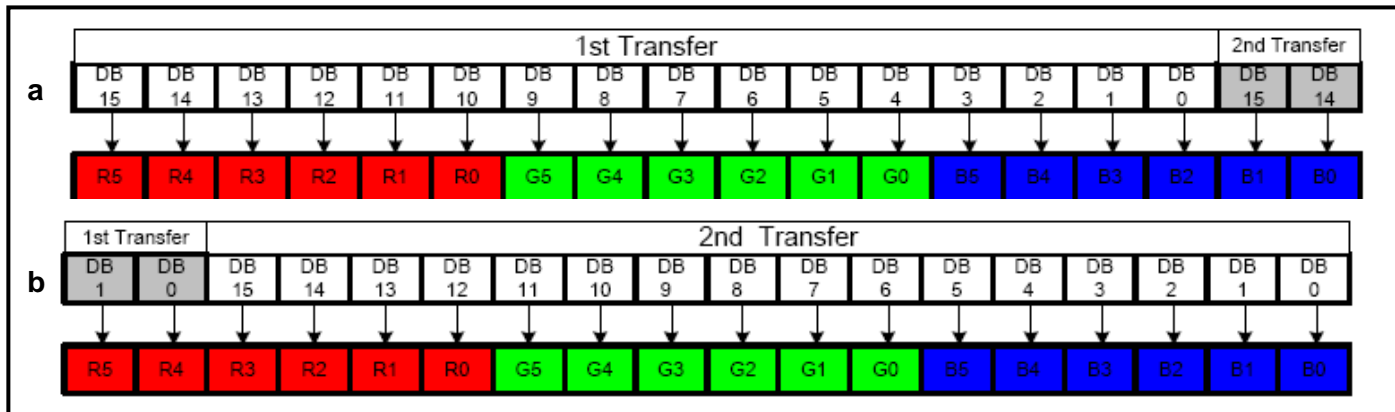
a. TRI=1,DFM=0,16+2-bit; b. TRI=1,DFM=1,2+16-bit;
